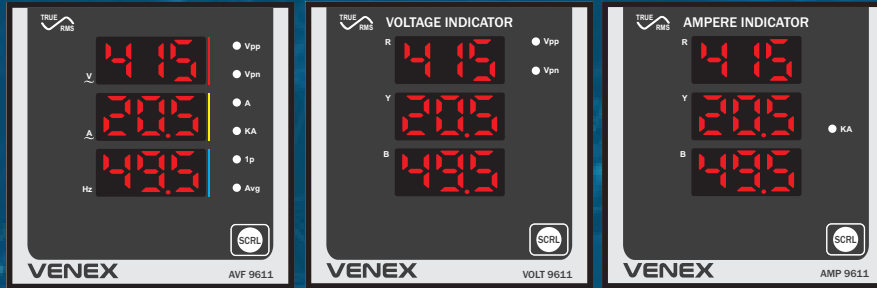
3 Phase Volt Indicator 3 Phase Amp. Indicator
